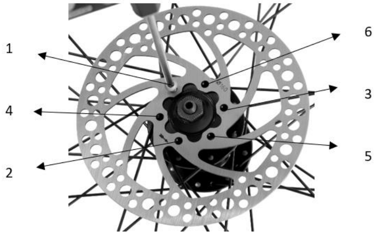
11. Atornillar los tornillos siguiendo el patrón de la imagen.
